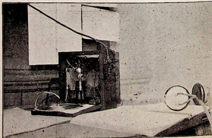
„Zak-ontvanger” waar vroeger PCGG op gehoord werd.
