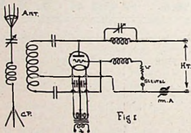
Hartley-schema.
